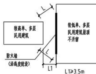
(b)相邻建筑高度不同的单、多层民用建筑平面图
