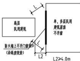
(b)高层民用建筑与单、多层民用建筑平面图
