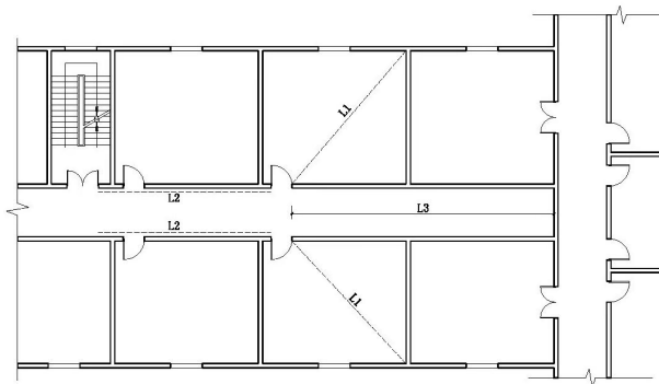
图示2:实际应用中，也确存在一些特例项目，端部的房间并没有向疏散走道开设疏散门（房间用作其他功能空间或通过其他疏散走道疏散），就可能出现L3较大的情况（图示2），这时应予以控制。 考虑L3走道部分的火灾危险性小于内部房间，因此，应参照“房间内任一点至房间疏散门的直线距离(L1)”，来控制L3部分的长度。以高层办公建筑为例，依《建规》5.5.17规定，图示2的L3距离，不应大于20m，当建筑内全部设置自动喷水灭火系统时，不应大于25m。
