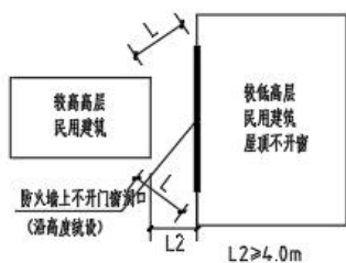
(a)相邻建筑高度不同的高层民用建筑平面图
