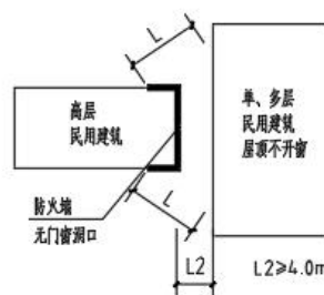
(c)高层民用建筑与单、多层民用建筑平面图
