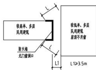
(a)相邻建筑高度不同的单、多层民用建筑平面图
