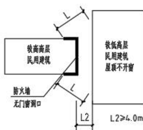
(b)相邻建筑高度不同的高层民用建筑平面图
