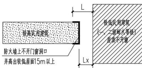
(b)情况二平面图
