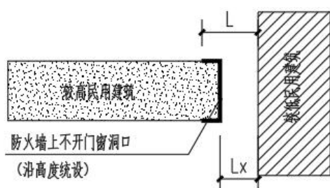
(a)情况一平面图
