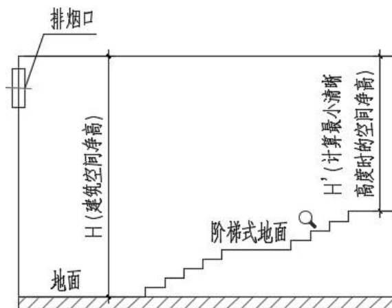
阶梯式地面场所 (侧墙排烟)
